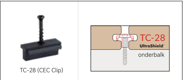
Standaard clips systeem
